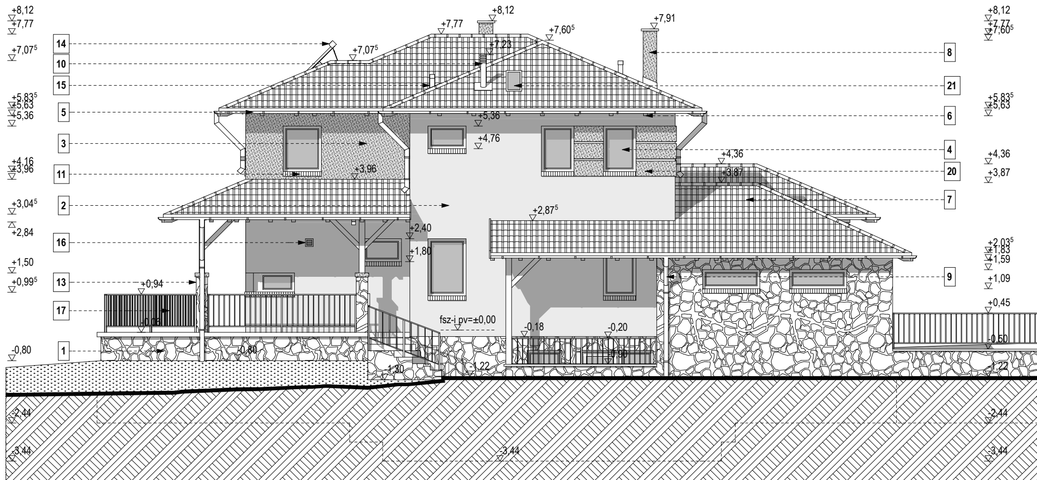
ÉSZAKKELETI HOMLOKZAT M 1:100
