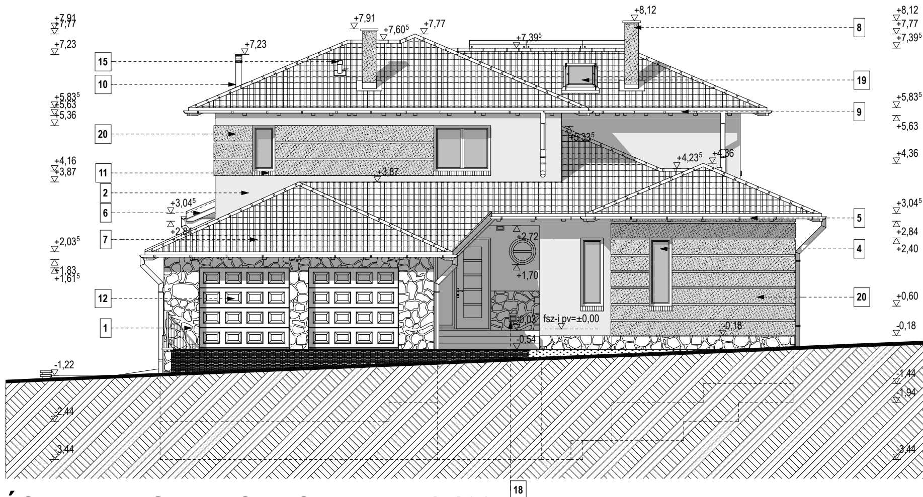
ÉSZAKNYUGATI HOMLOKZAT M 1:100
